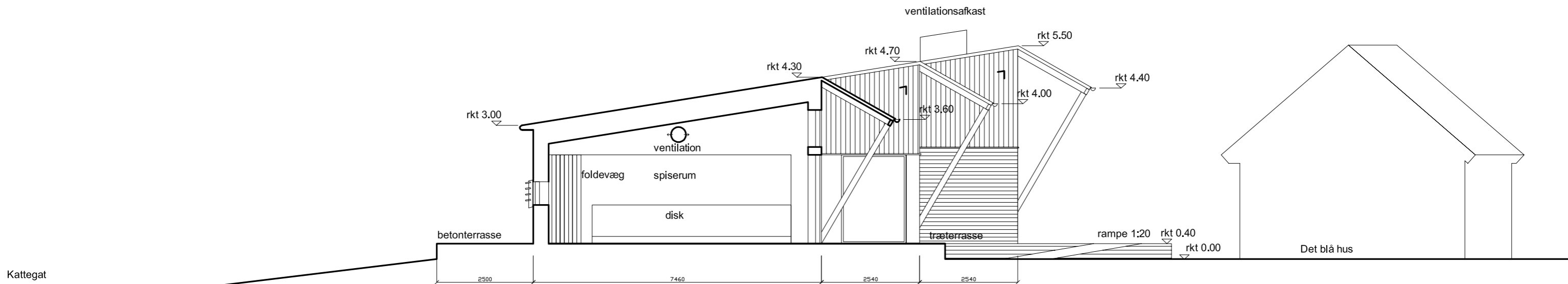
SNIT I SMAL DEL AF SPISEHUS 1:100 (i A3-print)
